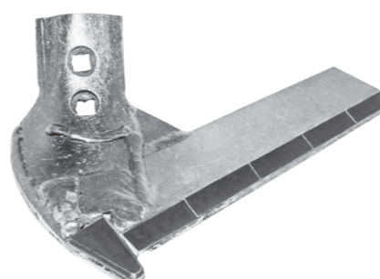
Rasette à plante type Boisselet
