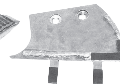
Soc Tarière type Boisselet
