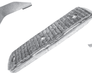
Patin broyeur type Egretier
